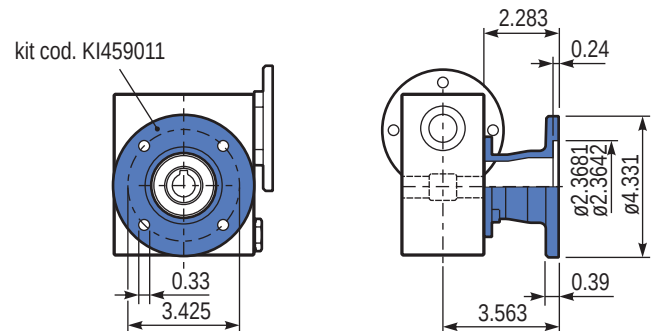
Single Shaft Albero lento semplice
