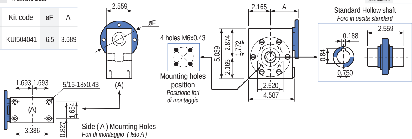
Modular base Base modulare
